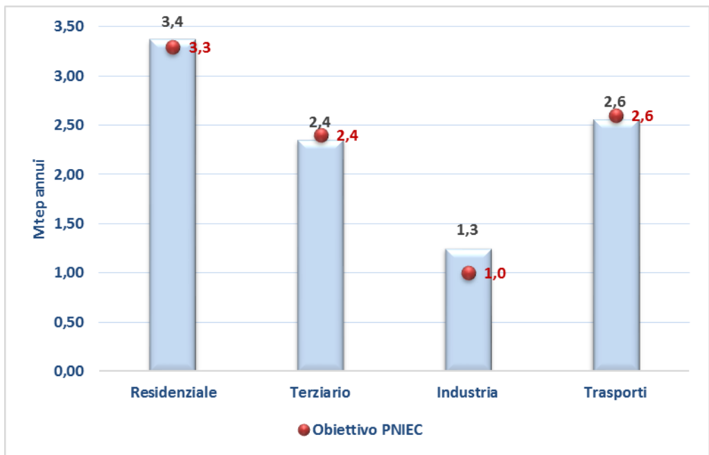
Figura 2: Obiettivo PNIEC al 2030
