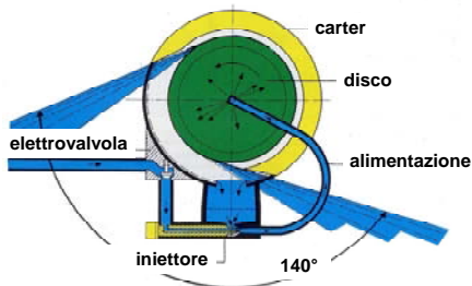
Fig. 192 - Esempio di ugello rotativo per barre irroratrici.
