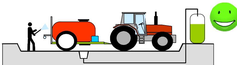
Fig. 92 - Area attrezzata per il lavaggio dell'irroratrice e per il convogliamento delle acque di lavaggio in appositi serbatoi di raccolta.
