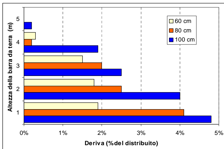
Fig. 50 – E' sempre opportuno mantenere l'altezza da terra della barra la più bassa possibile per ridurre la possibilità di deriva del prodotto fitoiatrice.
