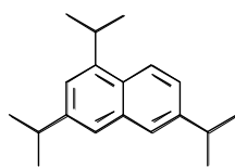
Ruetasolv TTPN
