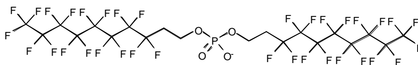
8:2 diPAP
