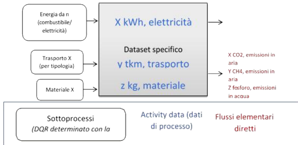
523 Figura 4. Rappresentazione grafica di un dataset specifico. Un dataset specifico del sistema in esame è un insieme di 524 dati parzialmente disaggregato: si deve valutare la qualità dei dati di processo (activity data) e dei flussi elementari 525 diretti. I valori di qualità dei sottoprocessi devono essere calcolati mediante la matrice DNM
