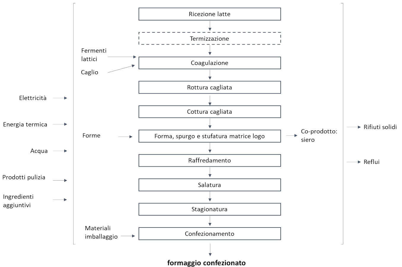
Figura 3. Fasi di lavorazione all'interno del caseificio
